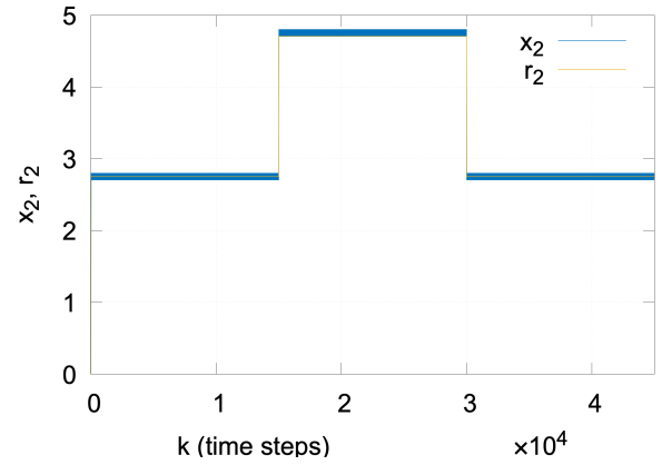
(d) C++, temperature x_2 .
